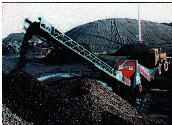
دپو ساز فله ای bulk depot unit
