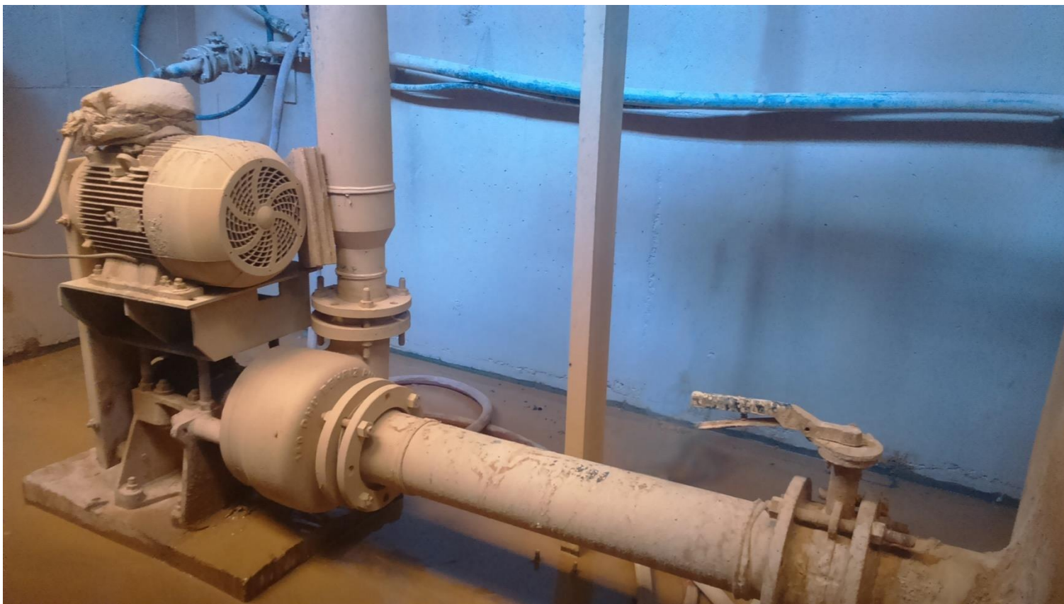
شکل ۲- پمپ اسلاری مدل SI-D-4-3 سرویس کاری : زیر فیلترپرس محل نصب: معدن سرب و روی دندی زنجان (کارفرما_کالسیمین)
