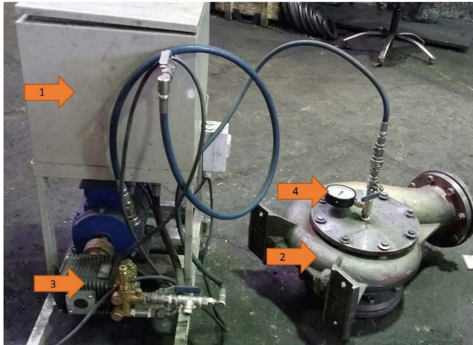
نمایی از تجهیزات تست هیدرواستاتیکی
